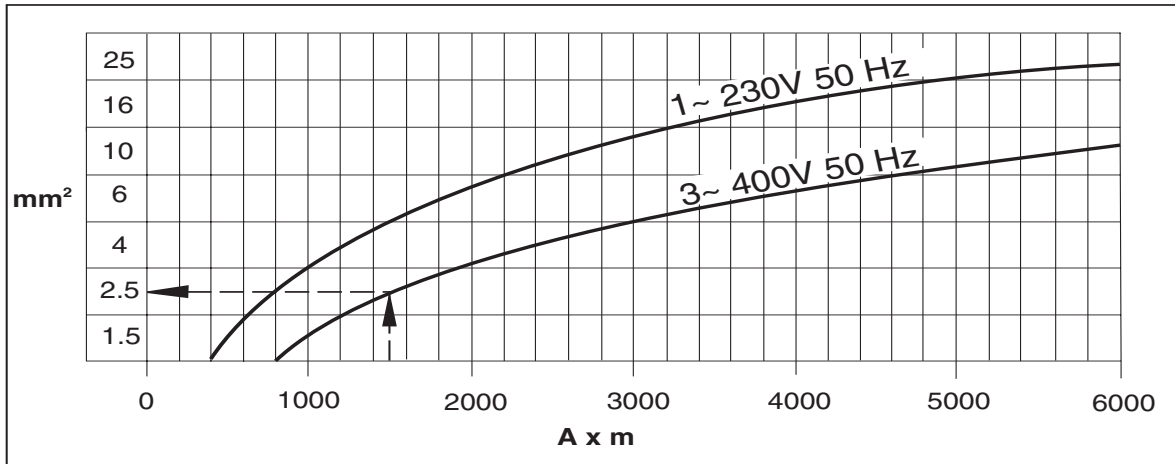
Minimum Uzatma Kablosu Boyutu Grafiği
